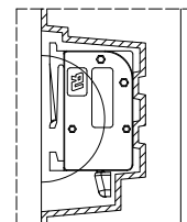
局部放大图B 比例5:1
