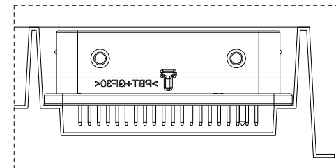
DETAIL: B 5:1
