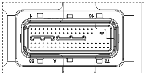
DETAIL: A 5:1
