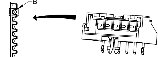
产品 比例 10 : 1
