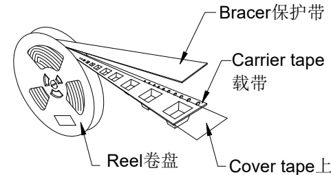
Material detail diagram 材料明细示意图
